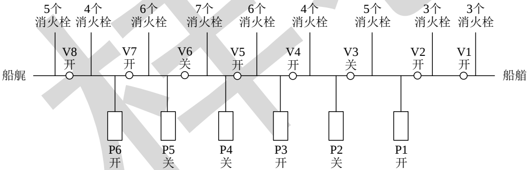
图 3 水消防管系图
