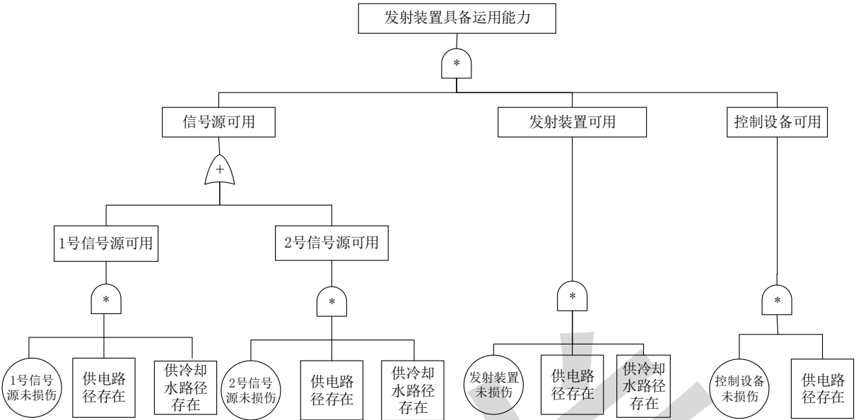
图 2 某发射装置具备运用能力的功能树
